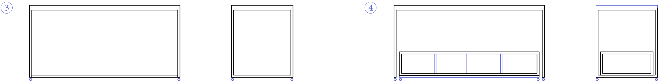
MESAS DE TRABALHO - introdução de rodas (3) e possibilidade de colocar as estruturas metálicas (2) por baixo (4)
