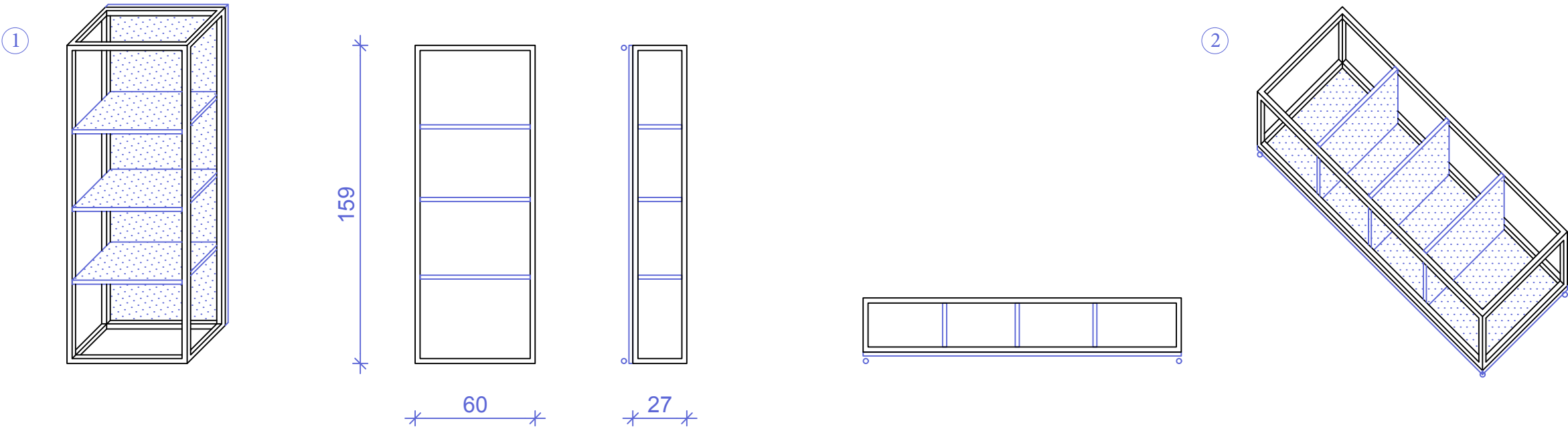
ESTRUTURAS METÁLICAS - introdução de fundo, prateleiras e rodas para posicionamento vertical (1) ou horizontal (2)
